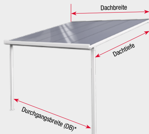
Modelle mit 3,06 m Dachbreite
